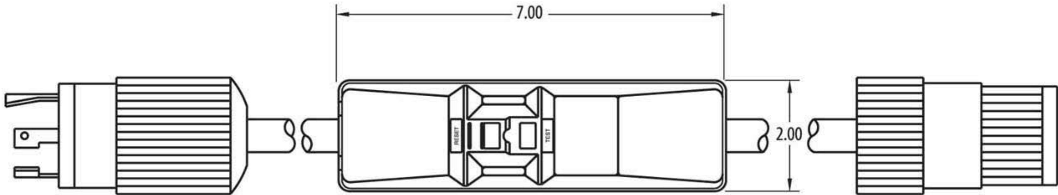
NEMA 5-30P TYP
