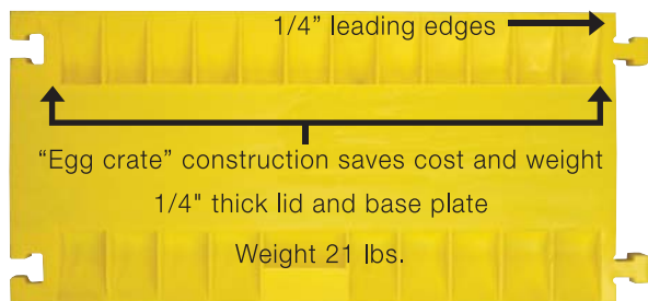
Cable Protector
