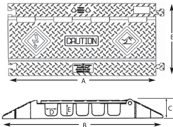
Cable Protector
